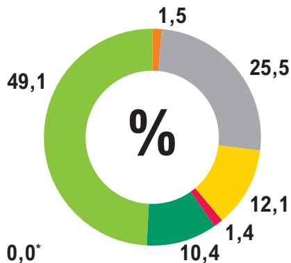
Energieträgermix Deutschland
